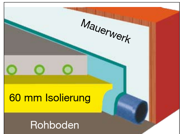
Verlegung des Rohrsystem auf dem Rohboden unter dem Estrich
