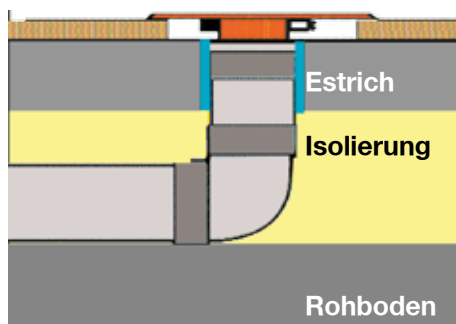
Bodendose in der Betondecke mit Estrich
