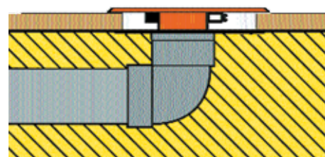
Bodendose im Dienboden
