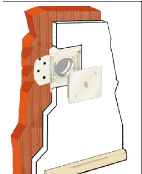
Einbaurahmen im Mauerwerk
