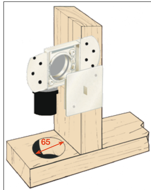
Einbaurahmen im Trockenbau
